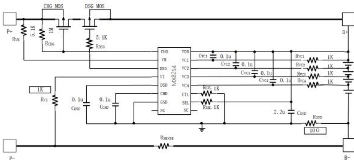
4串电池连接
