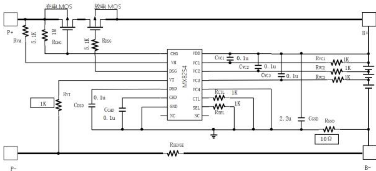
3串电池连接
