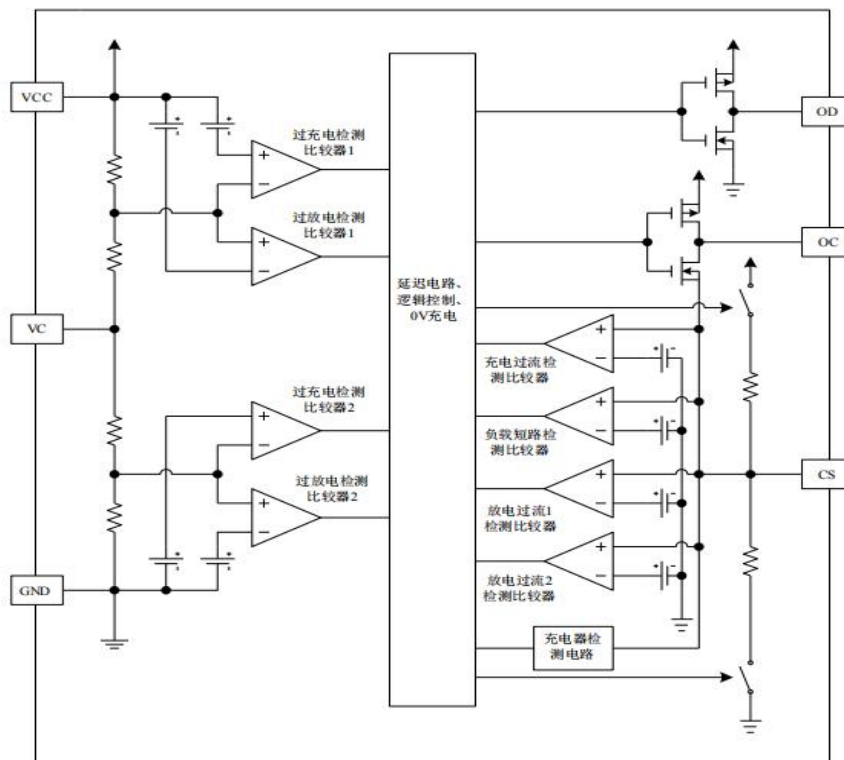
图 1 MX2122 系统框图
